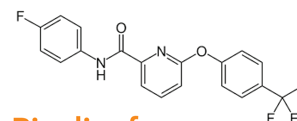
Picolinafen
