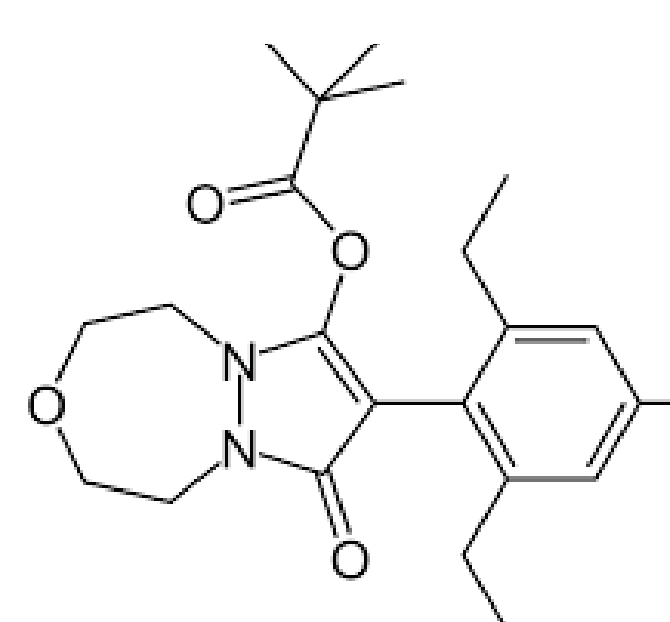
Pinoxaden
