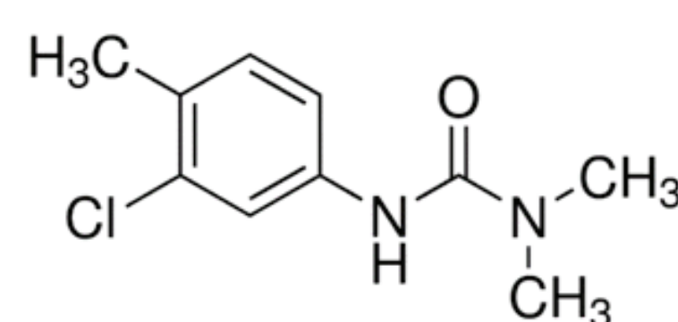
Chlorotoluron
