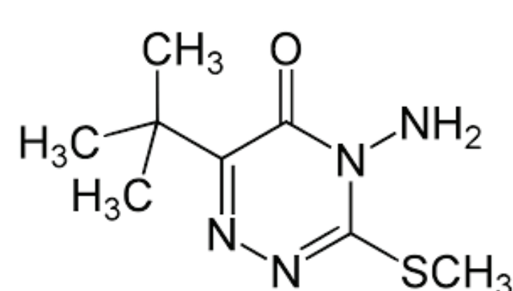
Metribuzin
