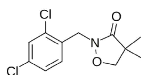
Bixlozone
