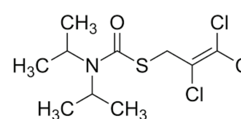
Tri-allate
