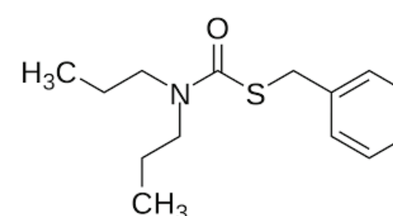
Prosulfocarb
