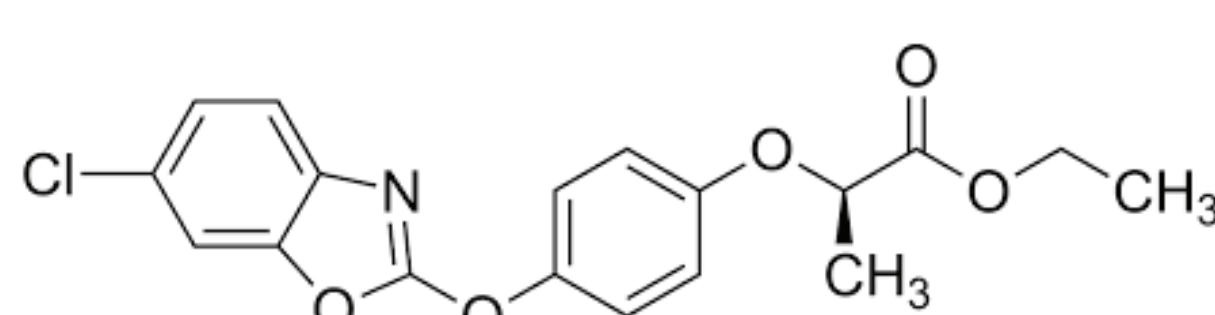
Fenoxaprop-ethyl
