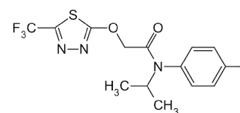
Flufenacet
